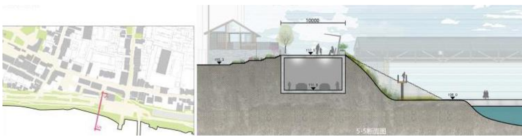
图 2. 拟设计下穿隧道与文星桥北位置关系剖面示意图
